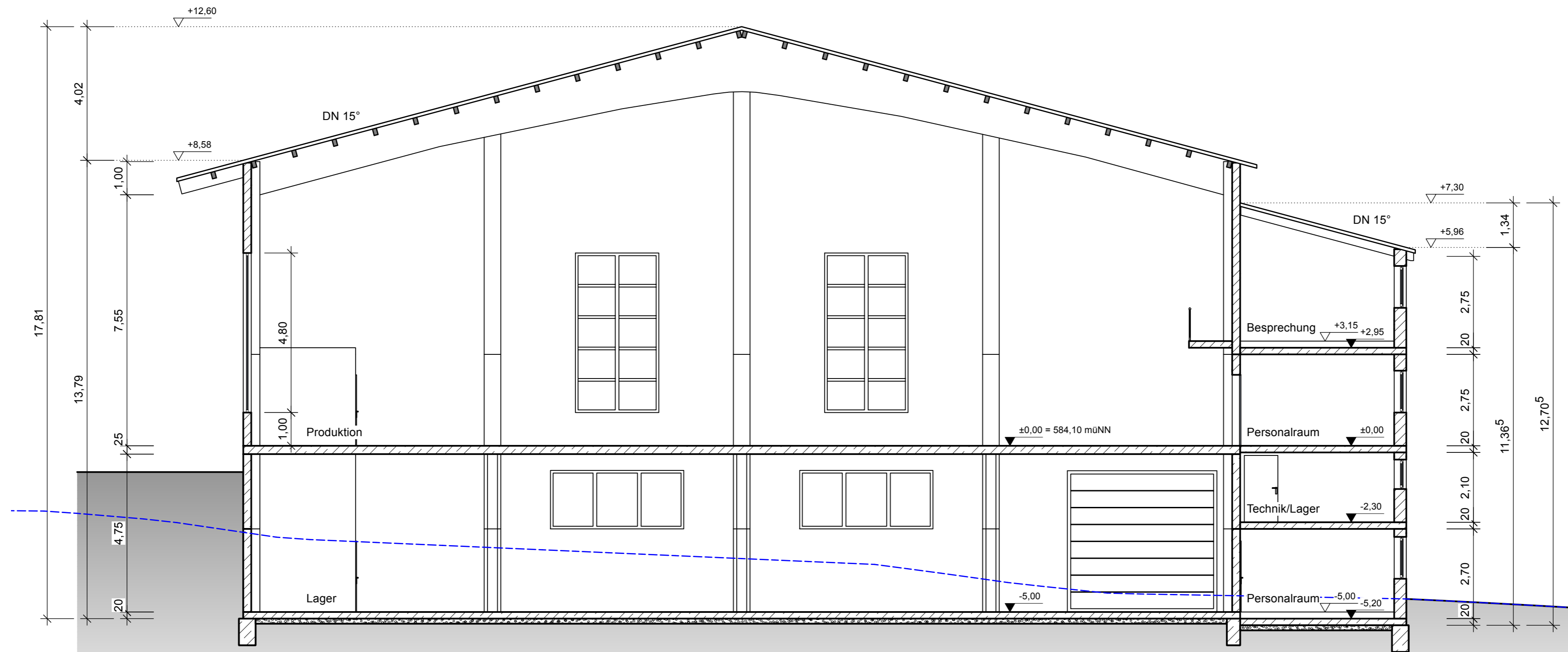
Schnitt A-A
