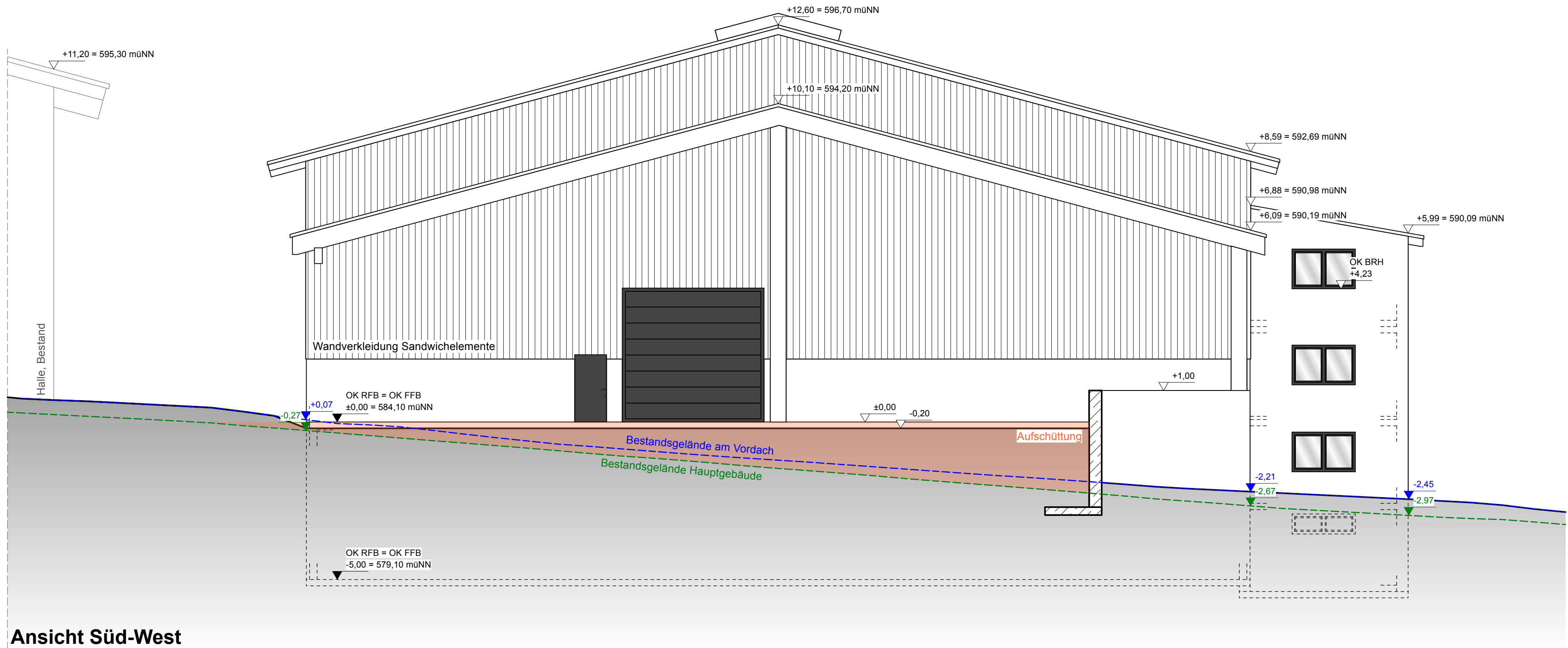
Ansicht Süd-West
